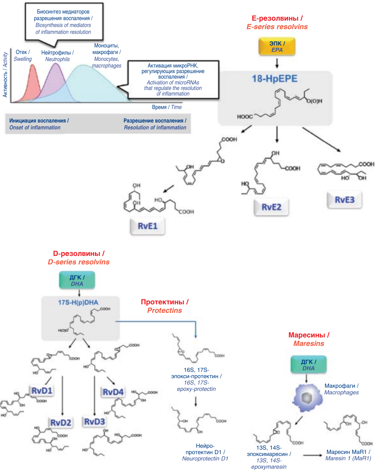
Рис. 1. Синтез химических медиаторов разрешения воспаления из ЭПК и ДГК (авторский рисунок). Fig. 1. Synthesis of chemical mediators of inflammation resolution produced from EPA and DHA (author's image).
