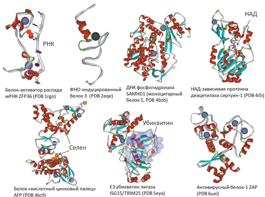
Рис. 4. Пространственные структуры цинксодержащих белков защиты от РНК-вирусов. Ионы цинка показаны в виде сфер.
