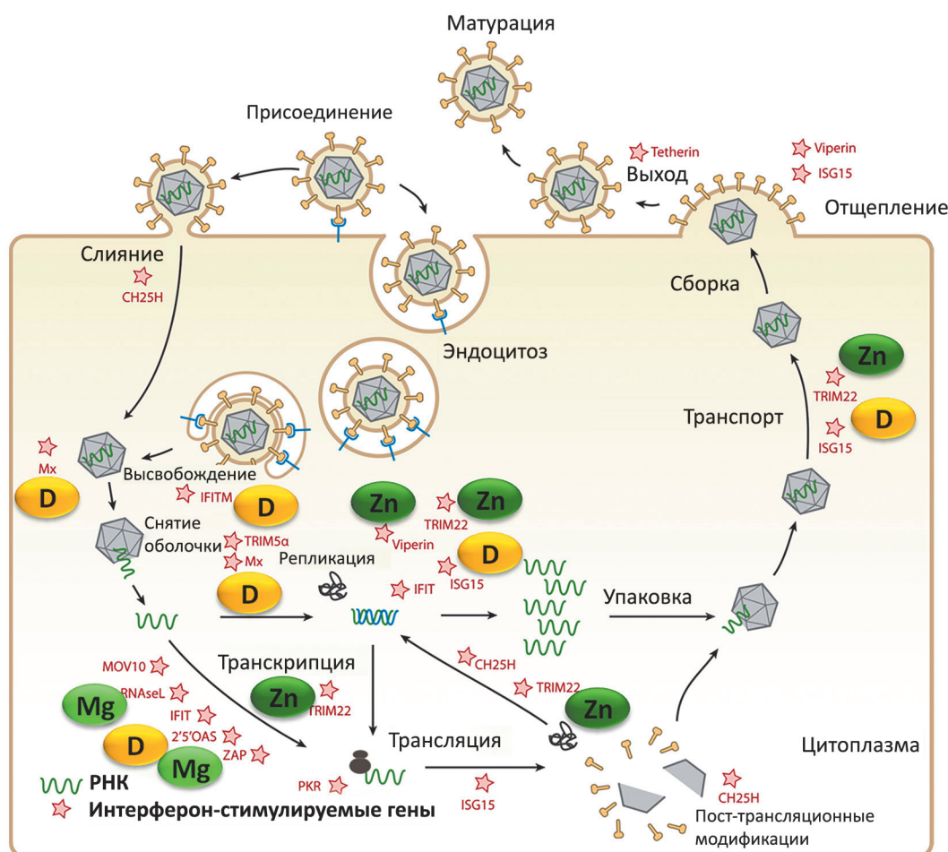
Рис. 2. Механизмы интерферонзависимой противовирусной защиты, жизненный цикл РНК-вирусов и соответствующие микронутриенты.
