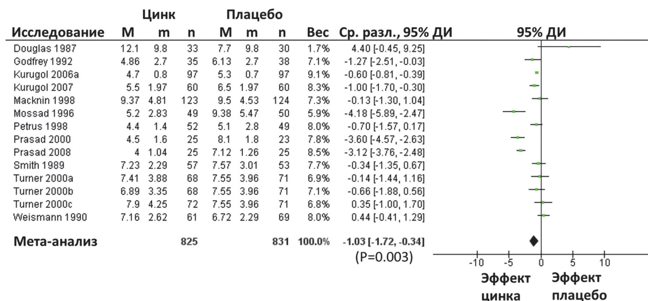
Рис. 5. Метаанализ исследований продолжительности симптомов ОРВИ при приеме цинка.
