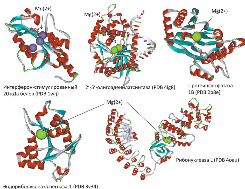
Рис. 3. Пространственные структуры магнийсодержащих белков защиты от РНК-вирусов. Fig. 3. Spatial structures of magnesium-containing protection proteins from RNA viruses.
